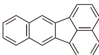
New Benzo[k]fluoranthene
